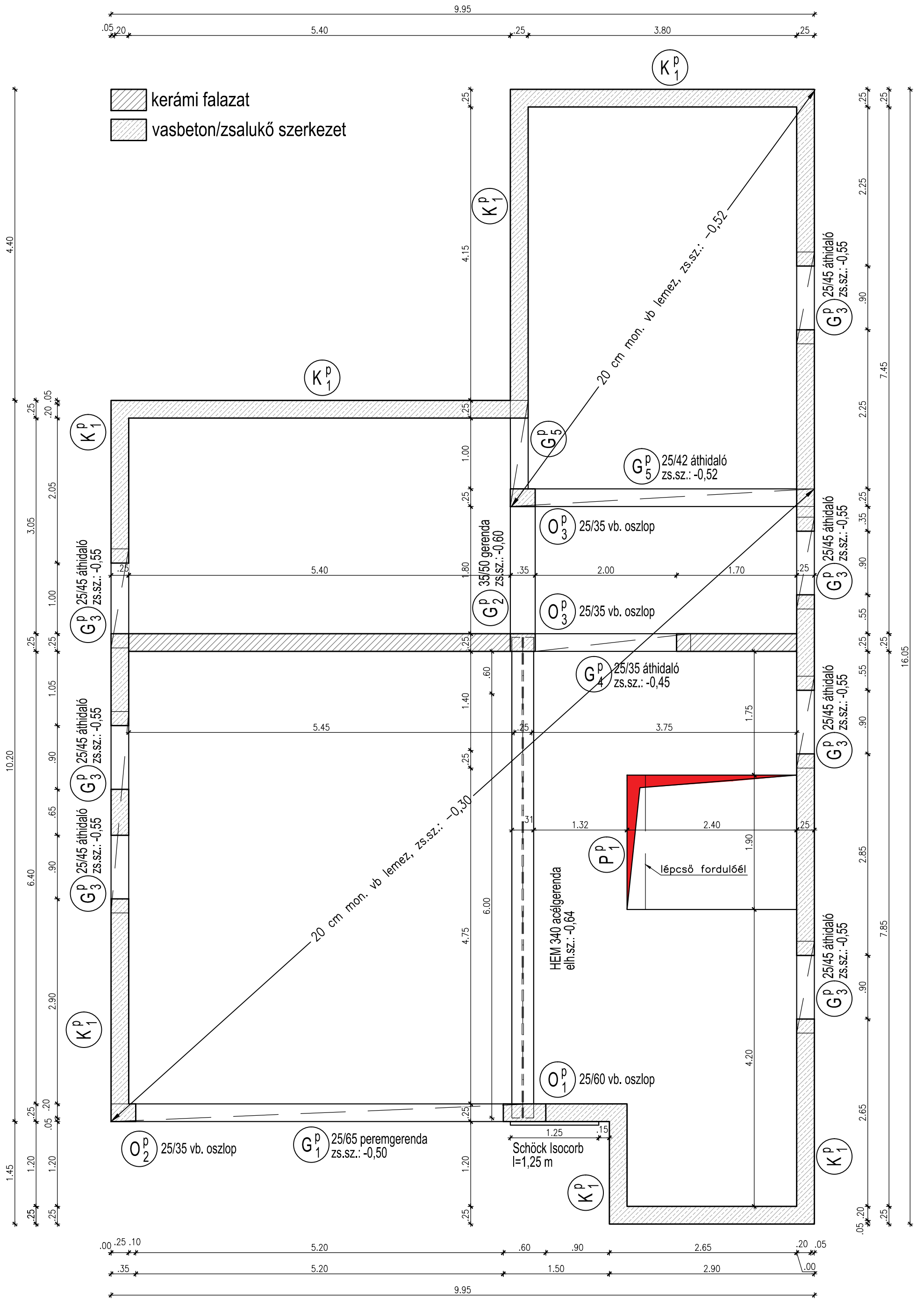
Pince feletti földem, M=1:50
